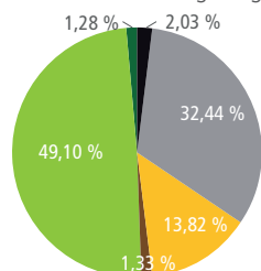
Verbleibender Energieträgermix
