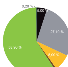
Verbleibender Energieträgermix
